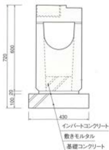
SK製品施工参考図
