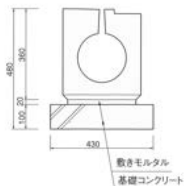
SK製品施工参考図
